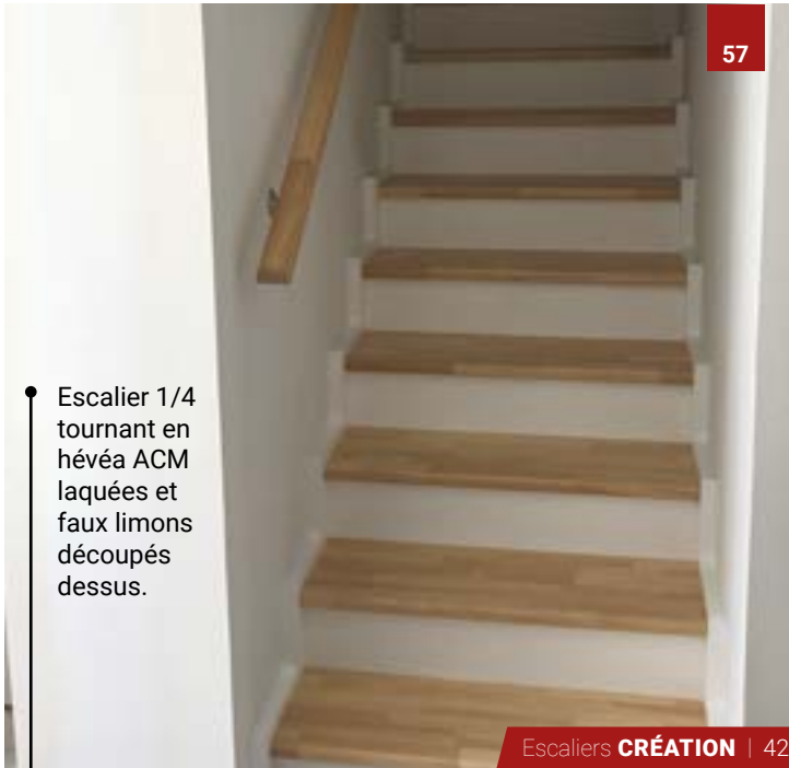
1/4 tournant avec main courante montée sur écuyers aluminium.
